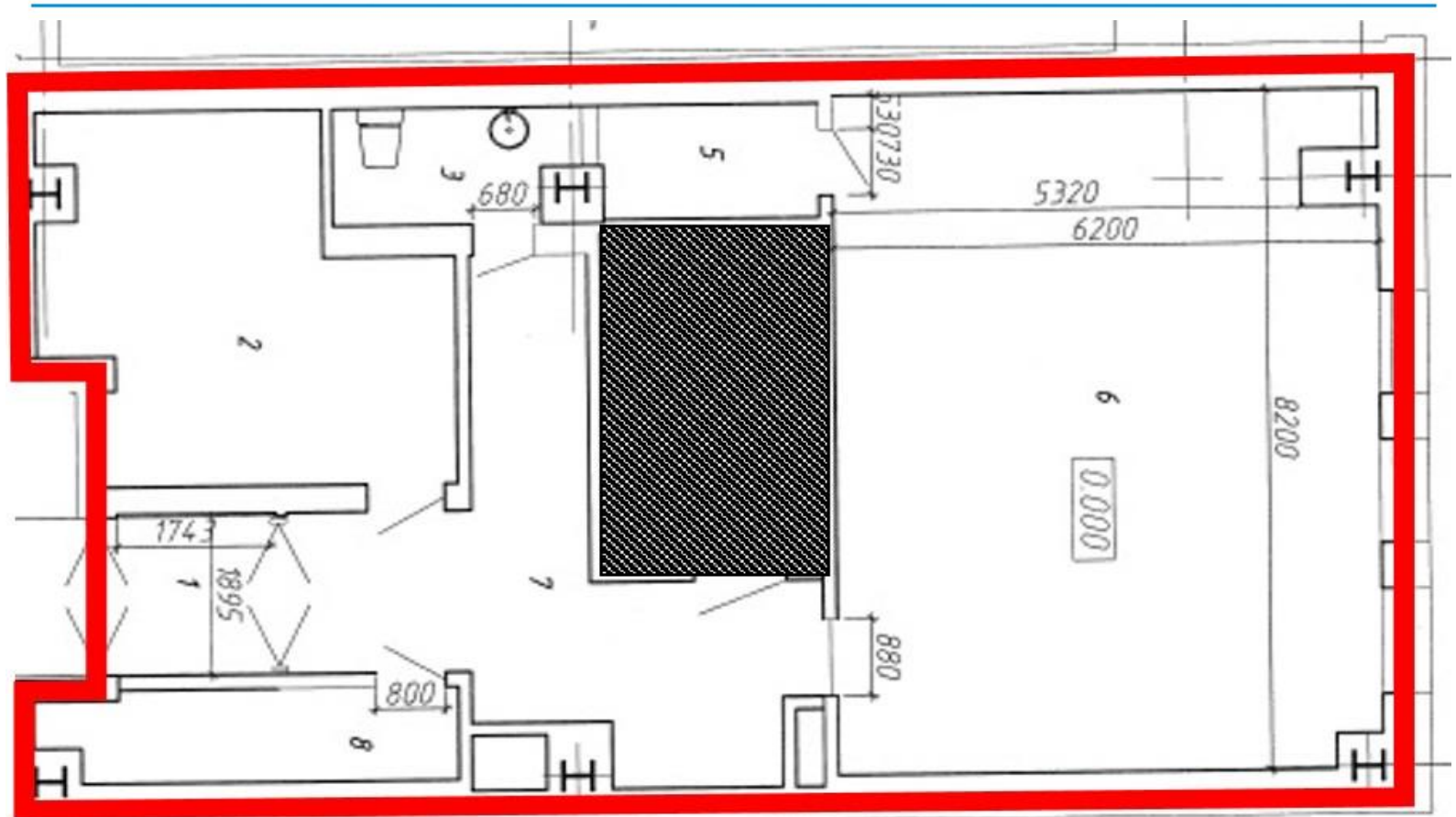
ПЛАН ПОМЕЩЕНИЯ
