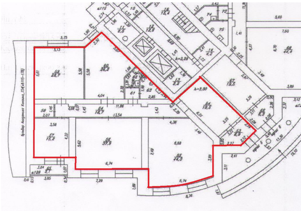
Рис. 3. План расположения помещений (объекта оценки)
