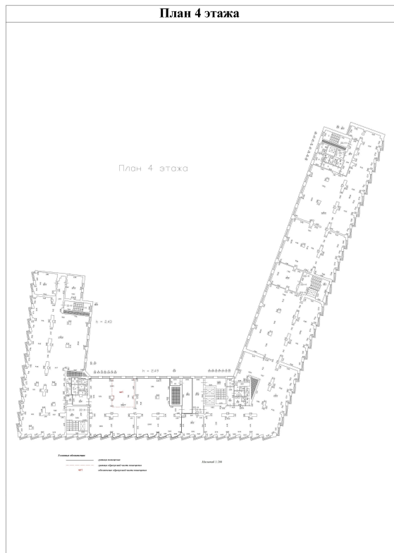
План 4 этажа
