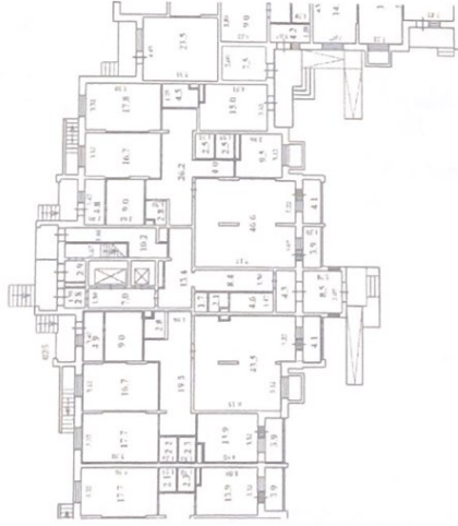
АС План части этажа 1 этаж 5 полвед
