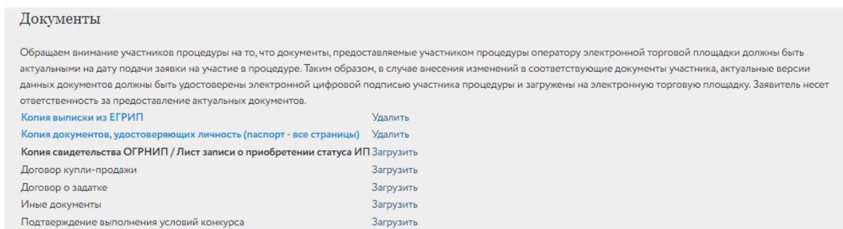
Рис. 8. Панель «Документы»
