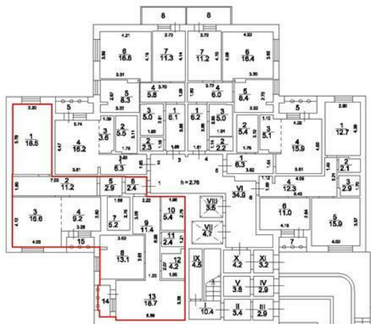
1 этаж
