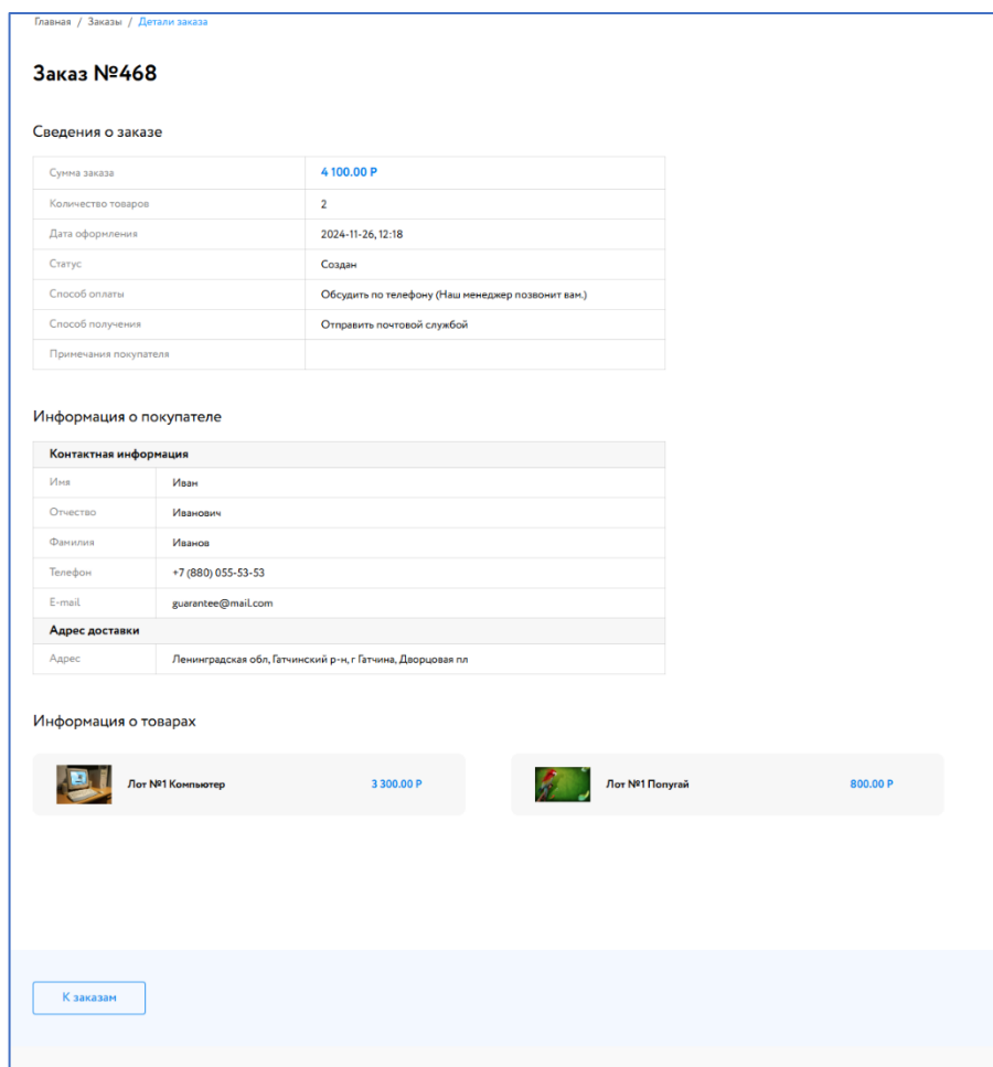
Рис. 15. Страница заказа
