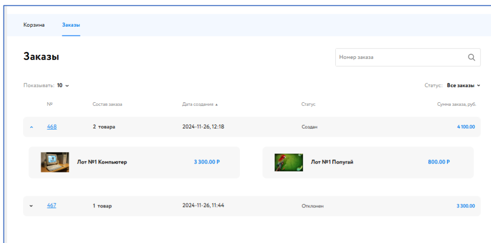
Рис. 14. Раздел «Заказы».
