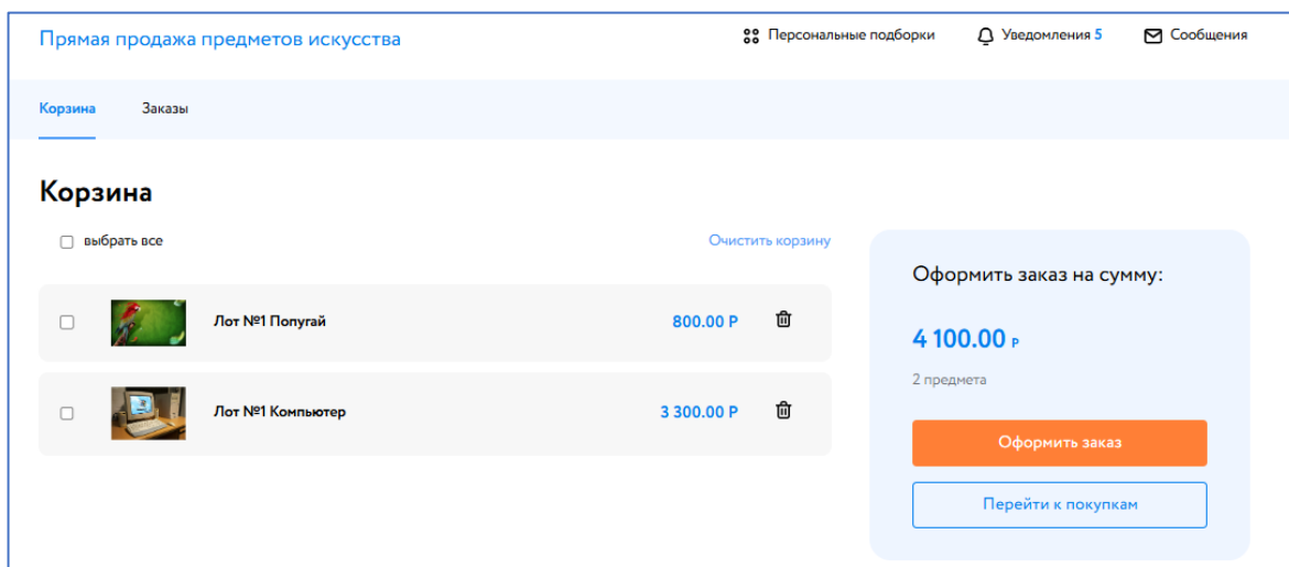
Рис. 11. Раздел «Корзина».
