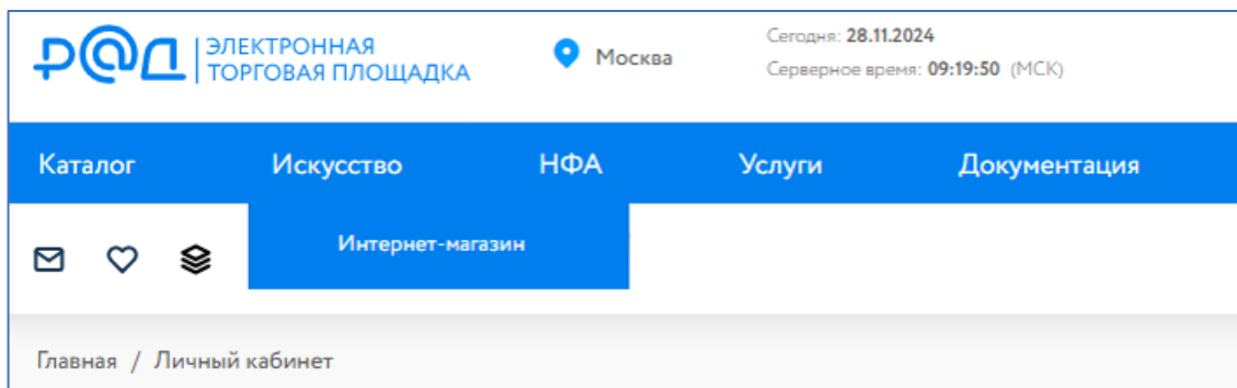
Рис. 1. Раздел «Интернет-магазин»
