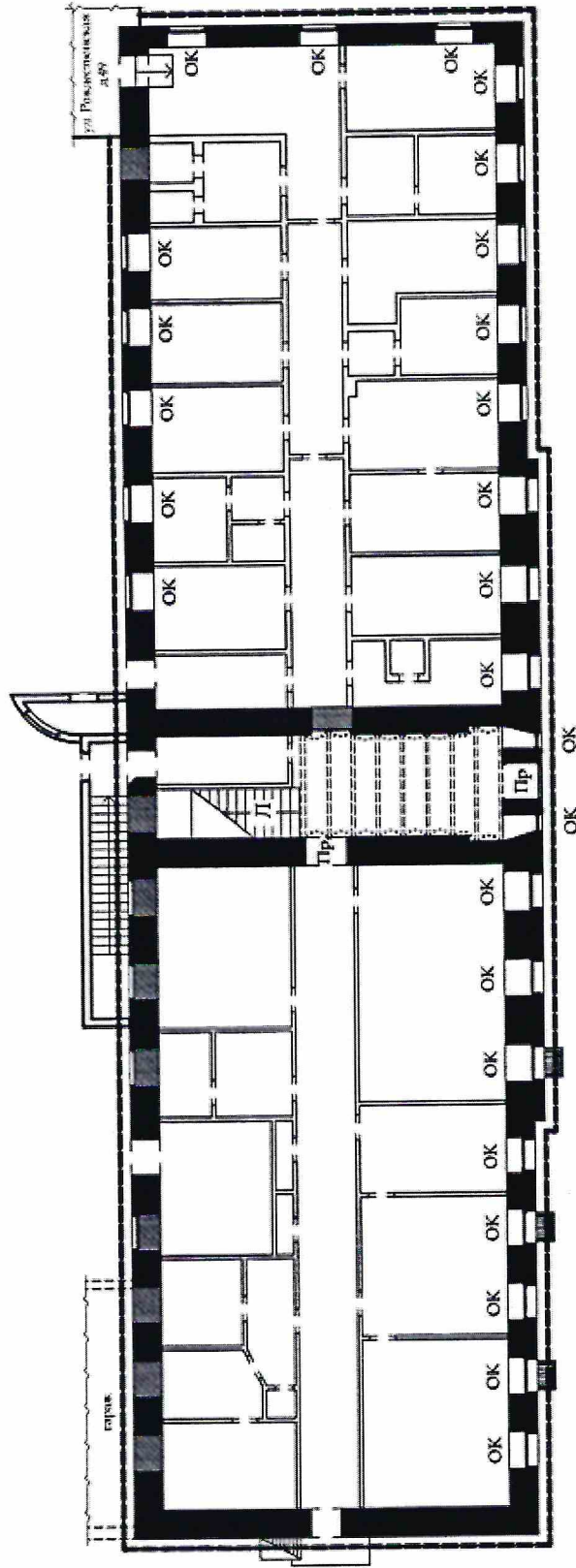
План первого этажа
